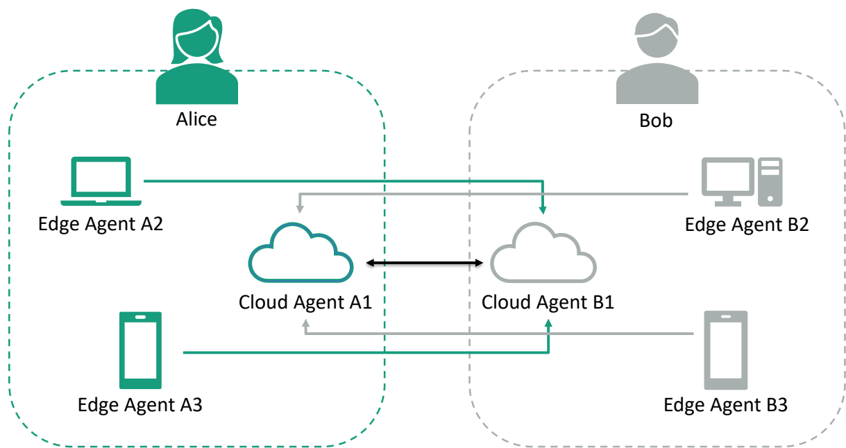
Abbildung 9: Agent-zu-Agent-Kommunikation
